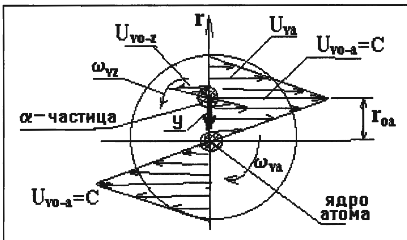
Рис.15.1 Пролет \alpha -частицы мимо ядра атома.
