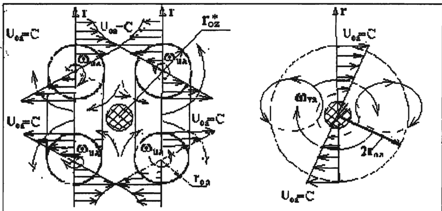
Рис.15.2 Схема протона
