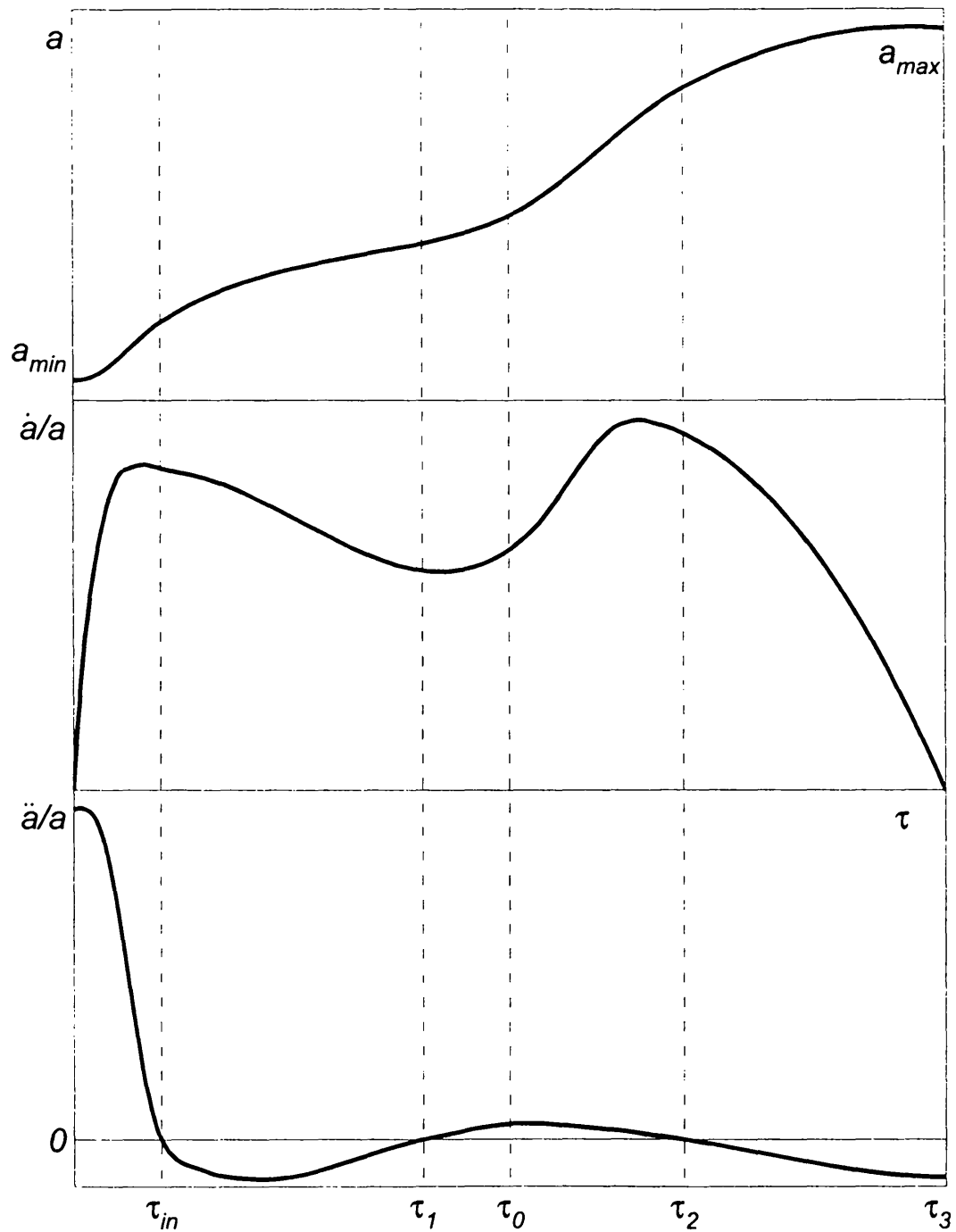
Рис. 1. Качественные кривые зависимости масштабного фактора, скорости и ускорения от времени \tau . Здесь \tau_{in} = 1,15\tau_T . Через \tau_0 обозначен современный момент времени.
