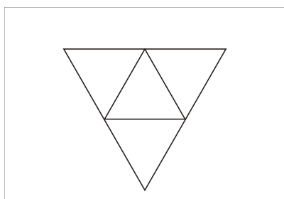
Рис. 1а. Соединение на плоскости четырёх треугольников.
