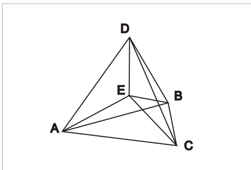
Рис. 2. Проекция четырёхмерной графемы-5 на гиперплоскость.
