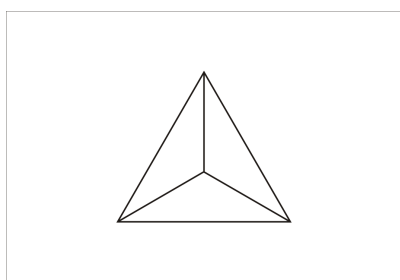
Рис. 1б. Соединение вершин в третьем измерении и проекция тетраэдра на двумерный мир.
