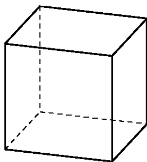
куб
