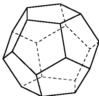
додекаэдр
