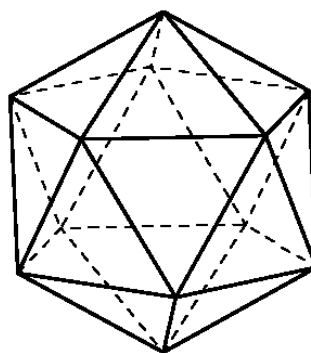
икосаэдр
