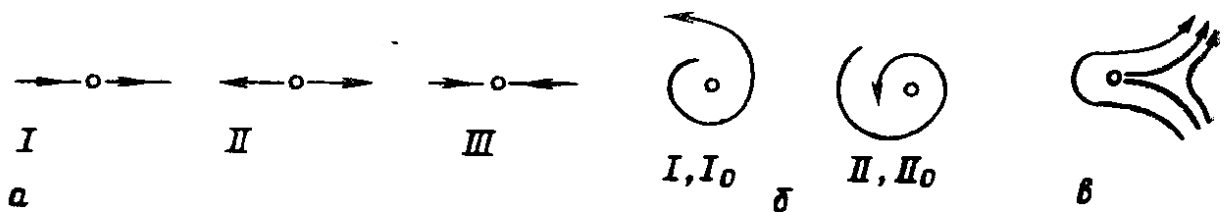
Рис. 13. Фазовые портреты векторных полей:
