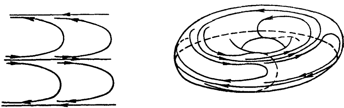
Рис. 10. Уравнение на торе без преобразования монодромии. Справа изображены фазовые кривые на торе, слева — фазовый портрет соответствующего двоякопериодического поля на плоскости.
