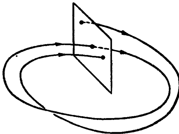
Рис. 5. Преобразование монодромии цикла.
