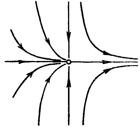
Рис. 16. Седлоузел.
