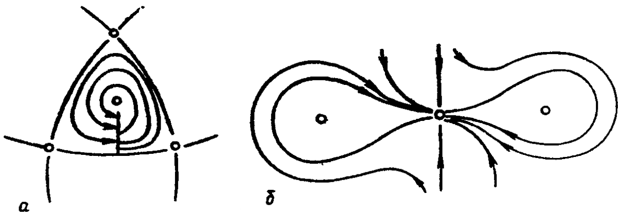
Рис. 20. Сложный цикл:
