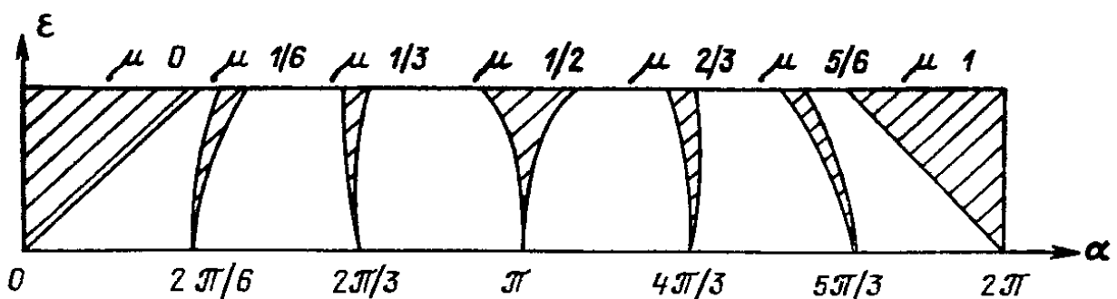
Рис. 11. Резонансные зоны для семейства диффеоморфизмов окружности.
