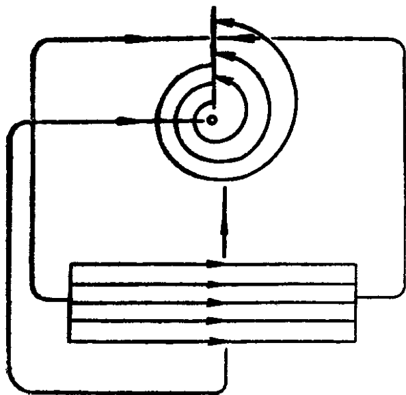
Рис. 17. Монодромная особая точка.
