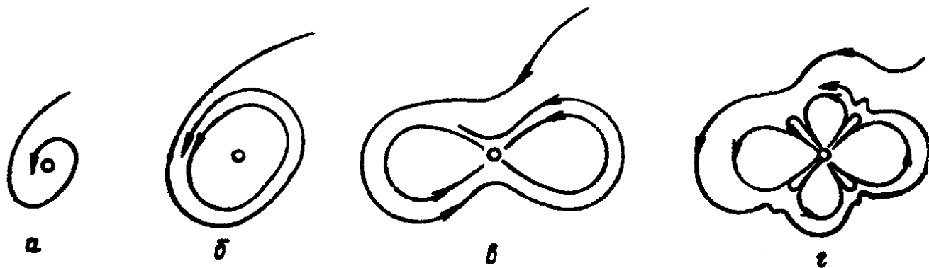
Рис. 7. \omega -предельные множества
