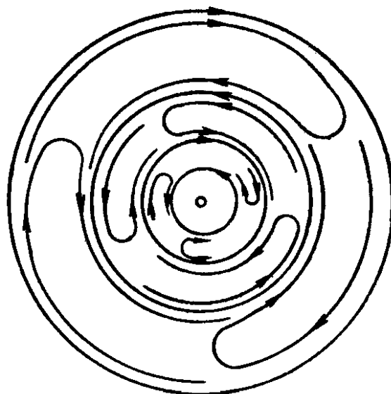
Рис. 18. Немондромная особая точка без характеристической траектории.
