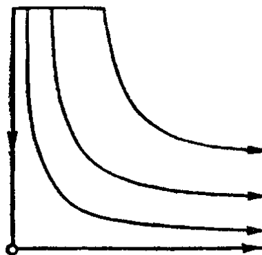
Рис. 21. Отображение соответствия гиперболического сектора.
