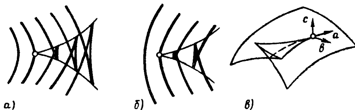
Рис. 9. Особая точка типа сборки складывания.
